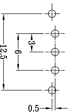
P.C.B LAYOUT
